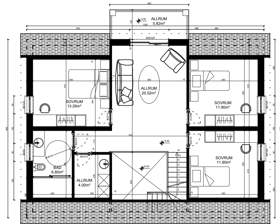
Indredningsbar Överplan 1:100
