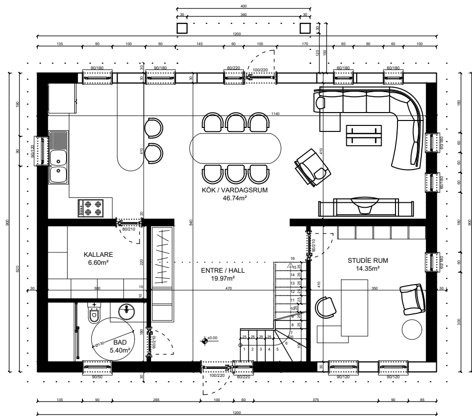
Entréplan 1:100
