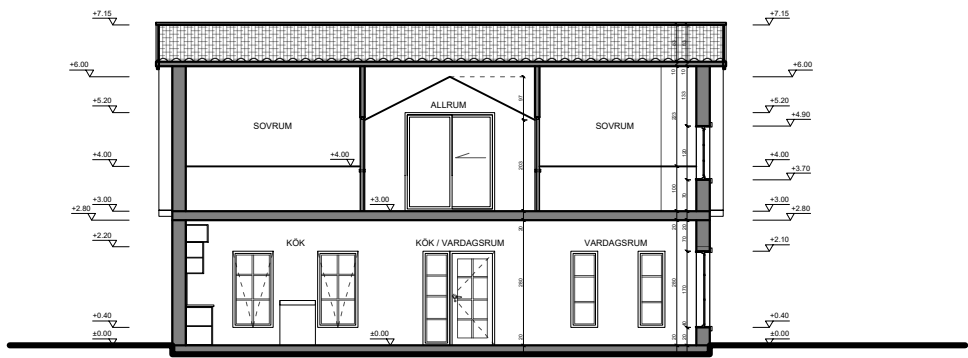
A-A SEKTION 1:100
