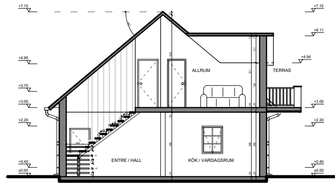
B-B SEKTION 1:100
