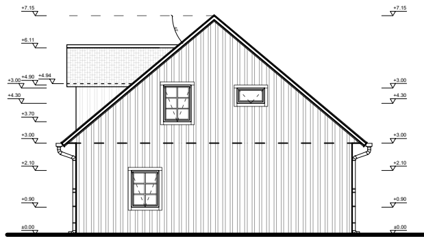
Högersida 1:100
