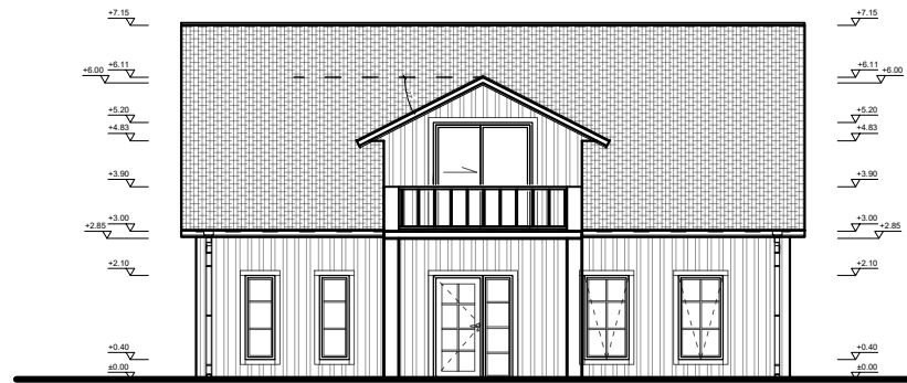
Baksida 1:100
